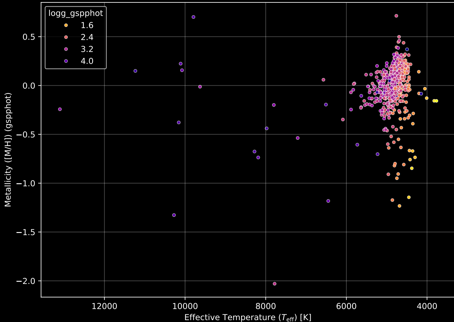
APOGEE DR17 Field: [064-06] Stellar Population Parameters (n= 544)
